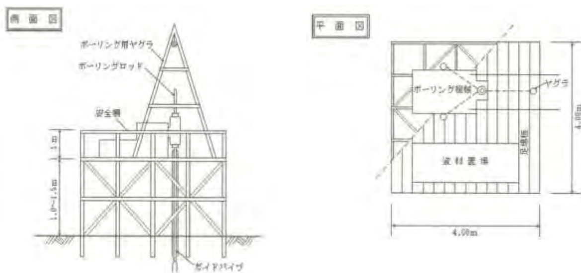
（嵩上げ足場）
