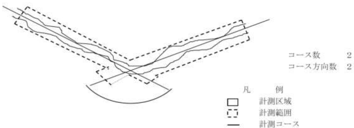
図 2-6-5 路線計測計画例 1
