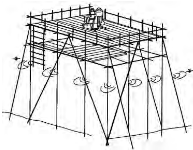
図 2-3-5 水上地足場概念図
