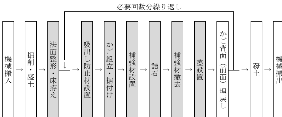
図 2-1 施工フロー
