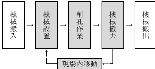
図 2-1 施工フロー
