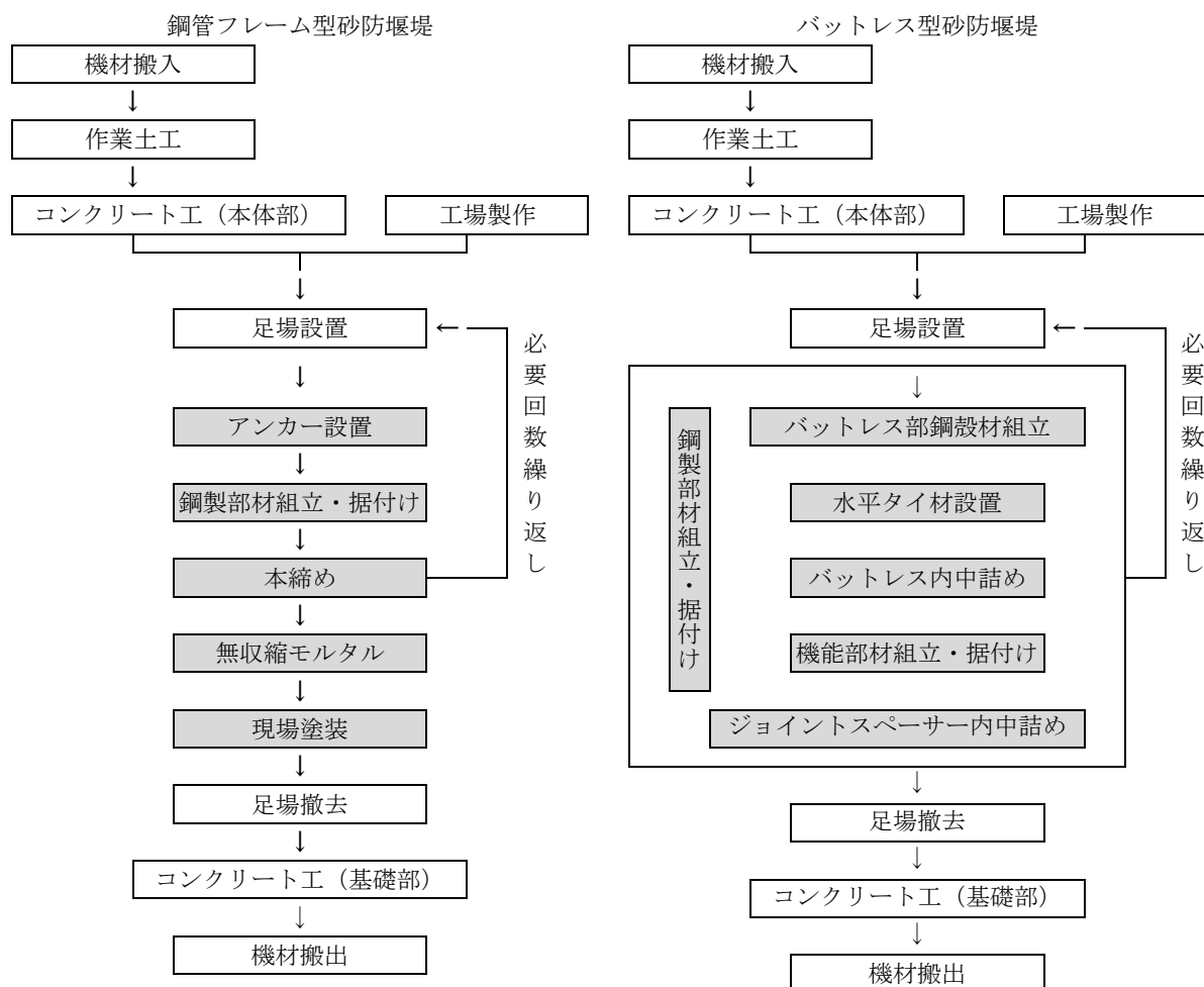
図 2-1 施工フロー
