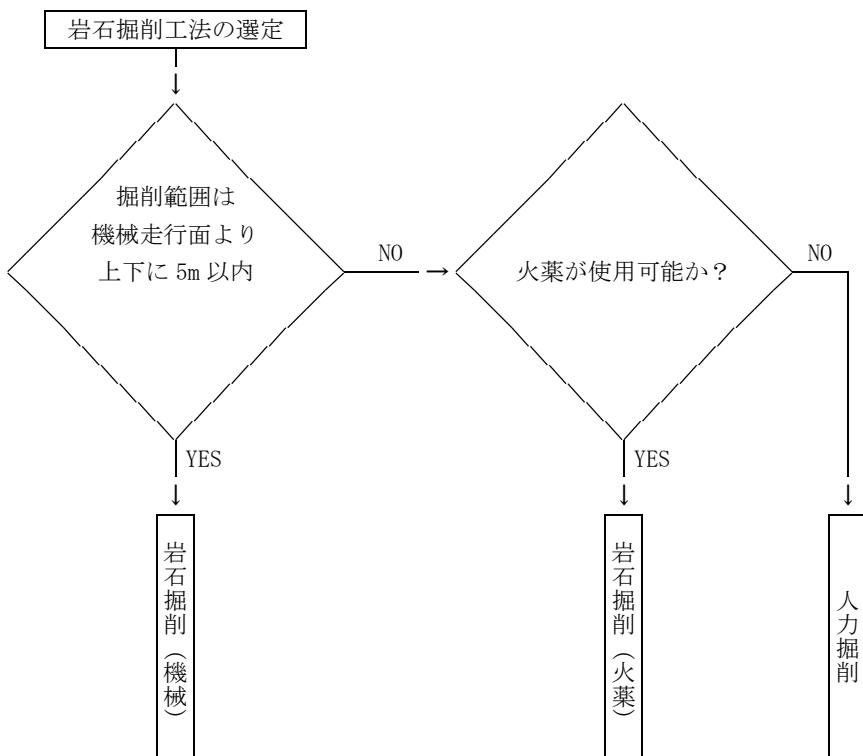
図 2-2 岩石掘削工法の選定
