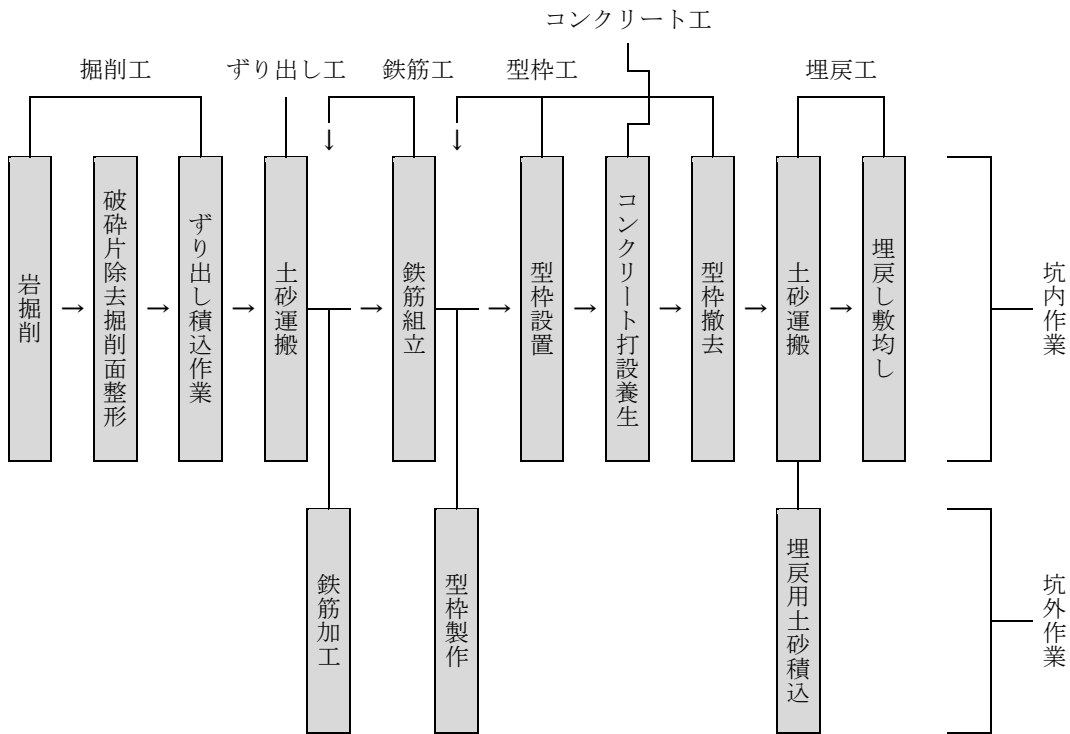
図 4.2 施工フロー
