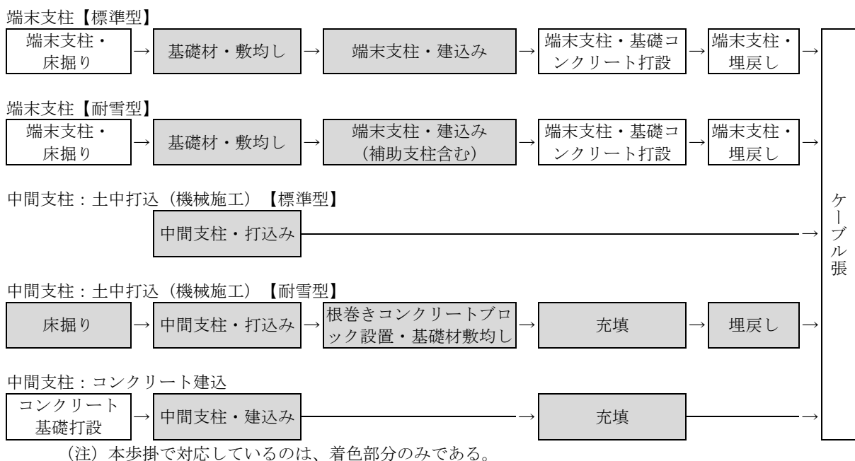
図 2-1 施工フロー
