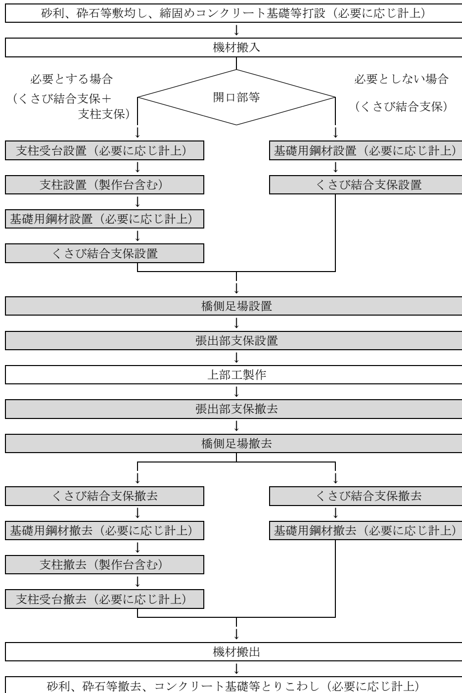
図 2-1 施工フロー
