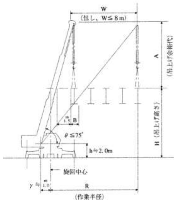
図 18.2 作業半径概略図/鈑桁（移動式クレーン油圧伸縮ジブ型）
