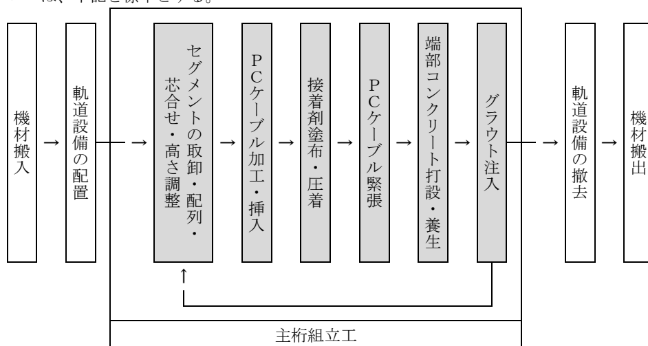
図 2-1 施工フロー
