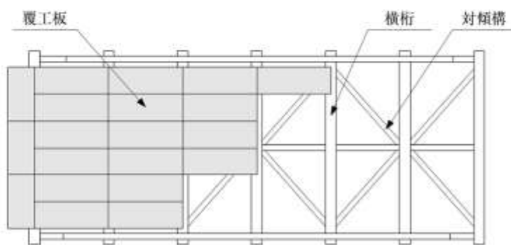
【平面図】
