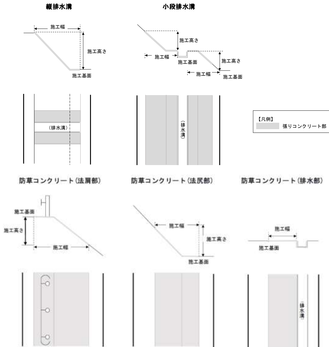
図 1-1 張りコンクリートの例
