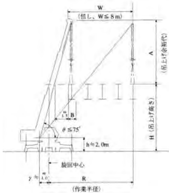
図 17.1 作業半径概略図/鈑桁（移動式クレーン油圧伸縮ジブ型）
