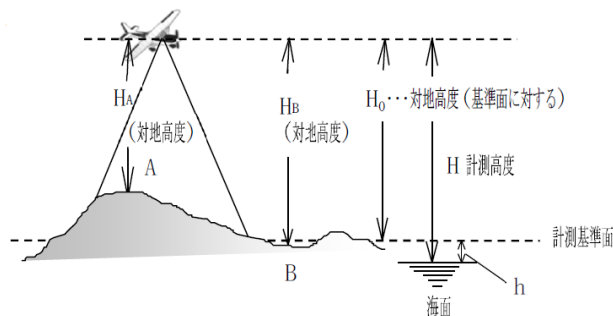
図 2-6-2 計測関係図
