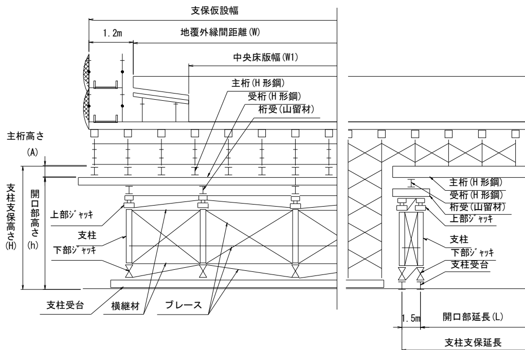
参考図（支柱支保工概念図（併用式））
