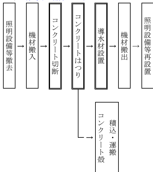
図 2-1 施工フロー（面導水）
