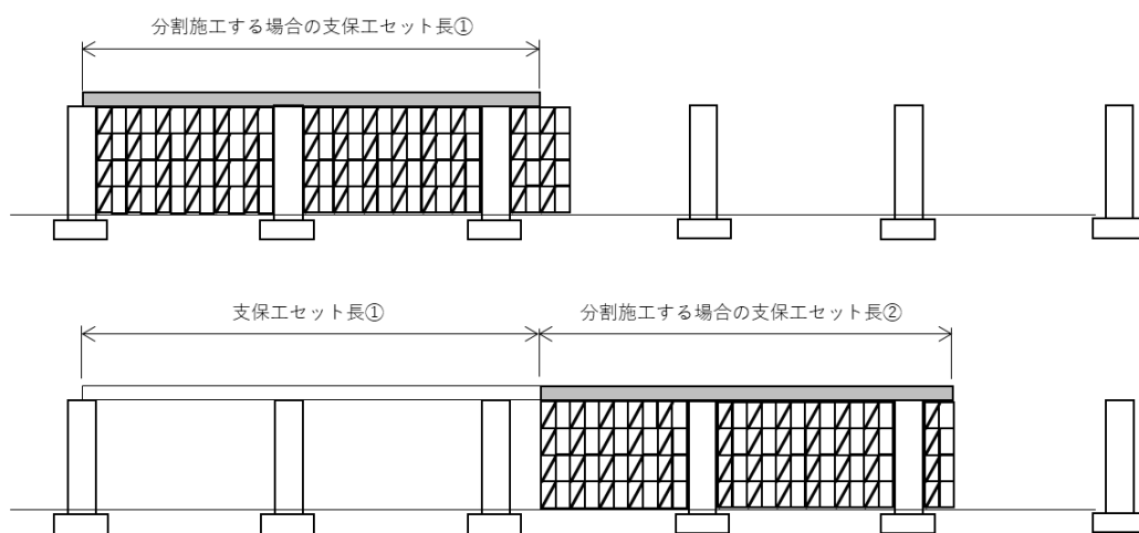
参考図（支保工セット長概念図）
