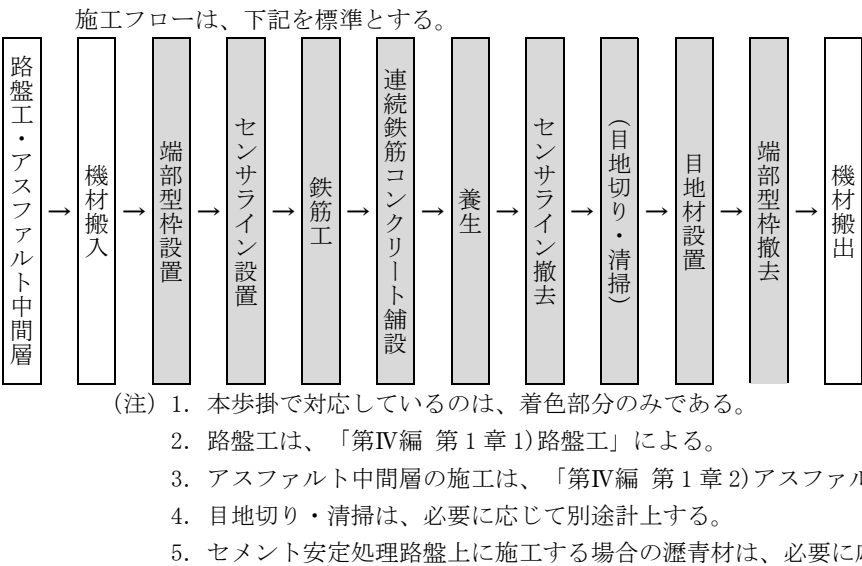
図 2.1 施工フロー
