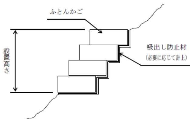
図 4-1 地すべり防止工（ふとんかご）概念図
