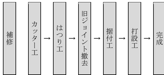
図 4-1 施工フロー（鋼フィンガージョイント等から既製品ジョイントへの取替え）
