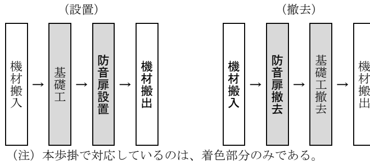
図 2-1 施工フロー
