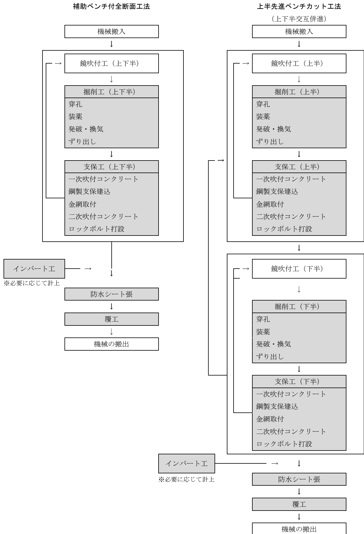
図 2-1 施工フロー
