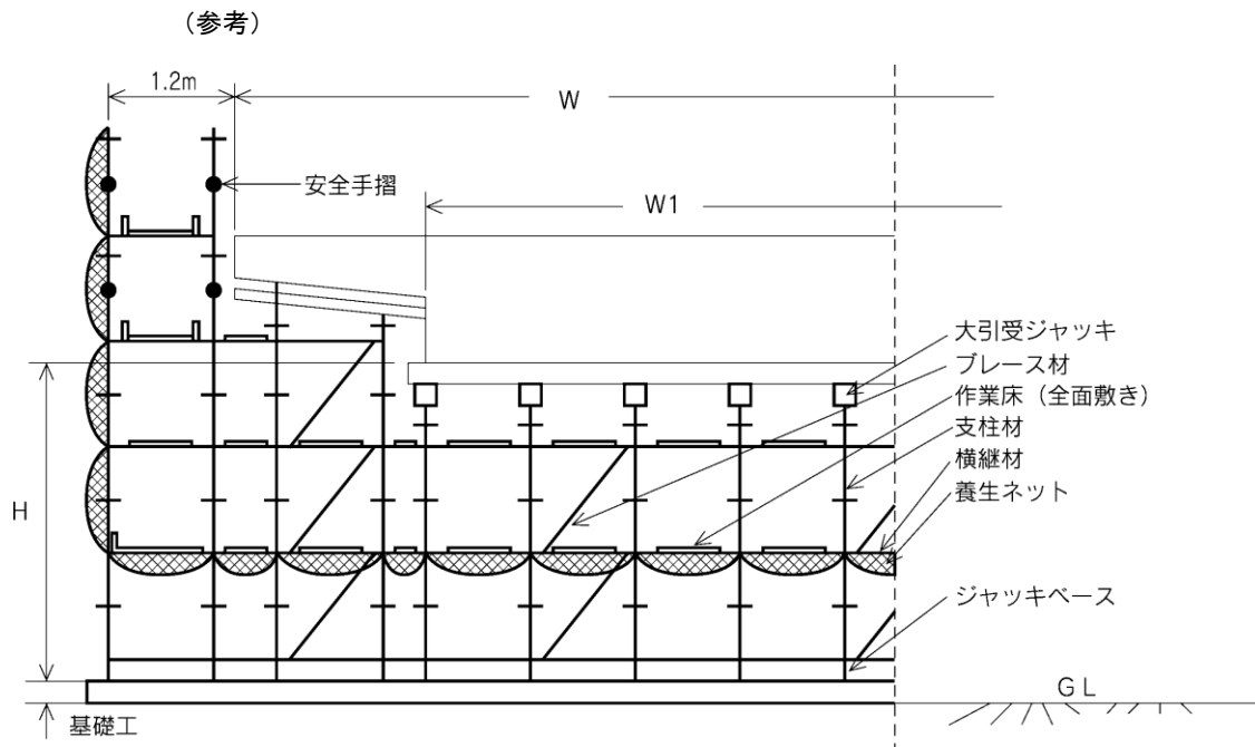
参考図（くさび結合支保工概念図）
