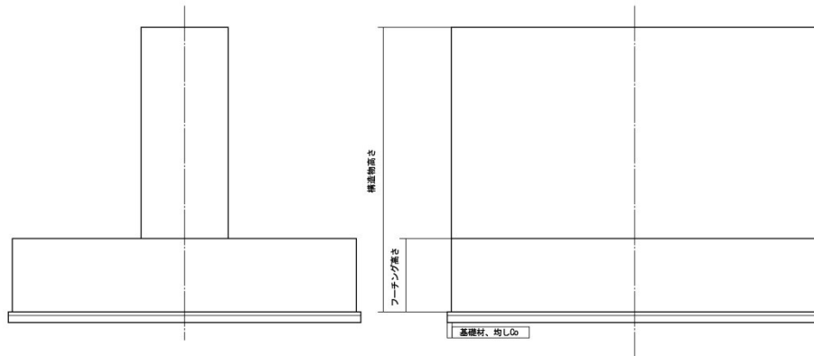
逆 T 式橋台
