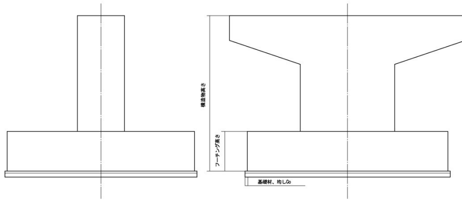
壁式橋脚
