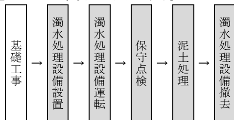
図 2-1 施工フロー
