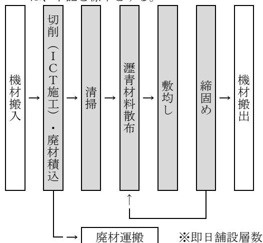
図 2.1 施工フロー
