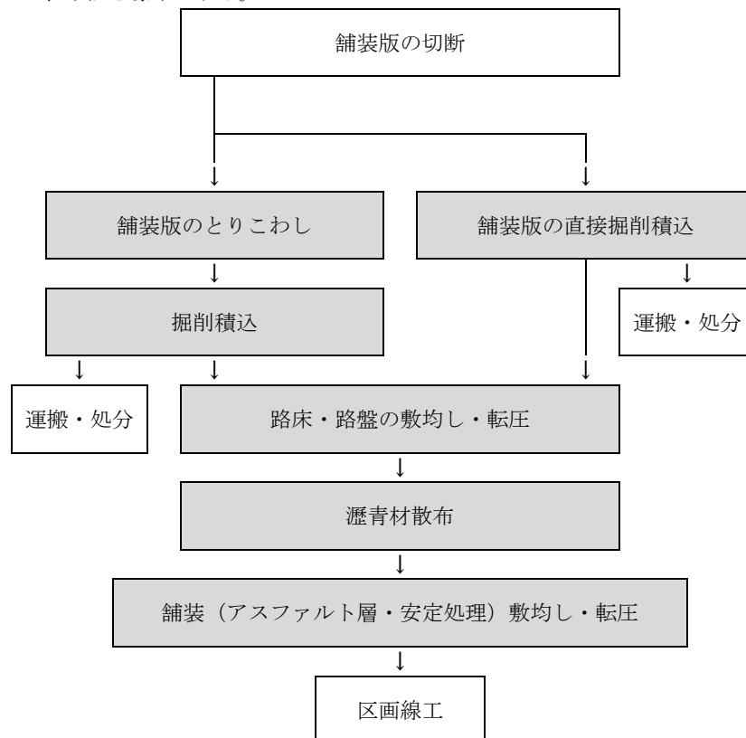
図 2-1 施工フロー
