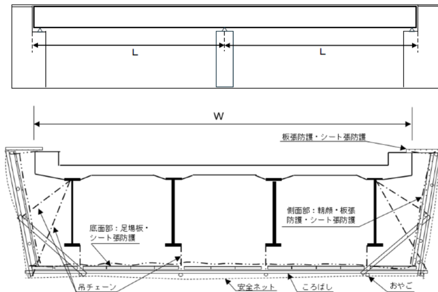
パイプ吊足場参考図
