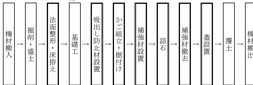
図 2-1 施工フロー
