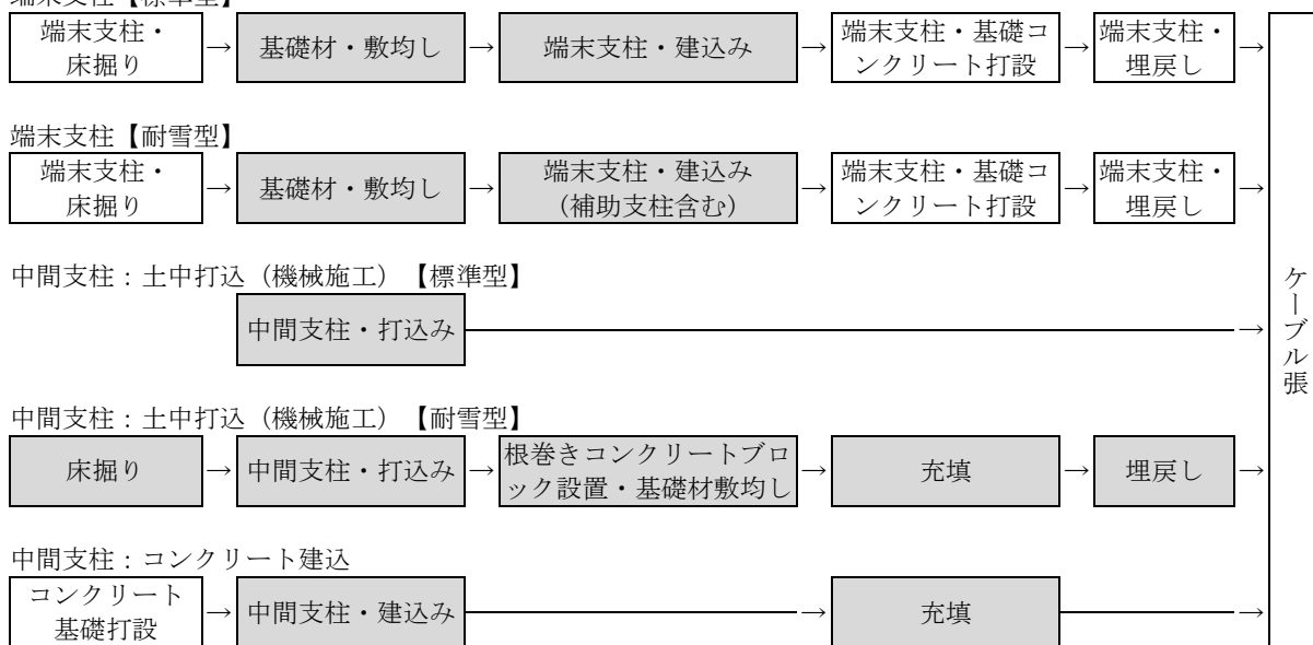
図 2-1 施工フロー
