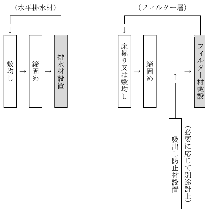
図 2-1 施工フロー
