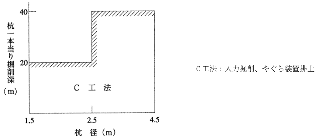
図 1-2 適用杭径及び掘削深（標準）
