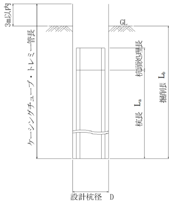
図 5-1 施工図
