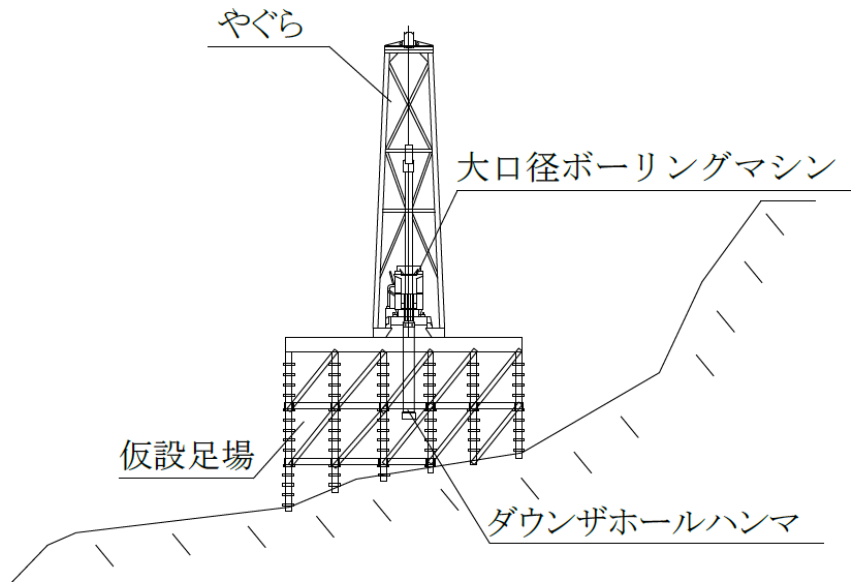
参考図 (B 工法模式図)
