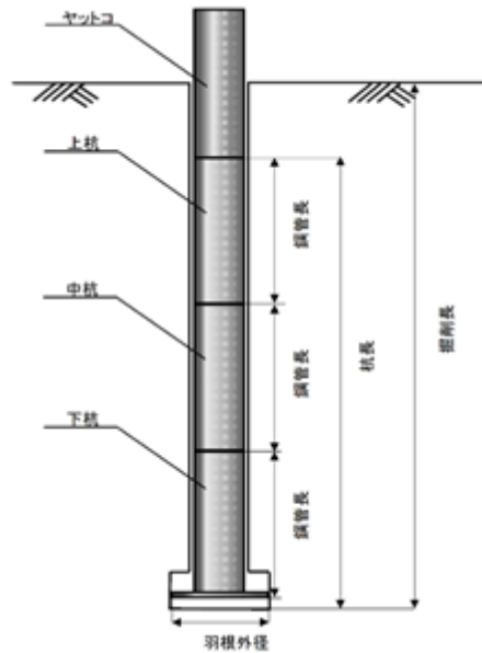
図 1-1 施工図
