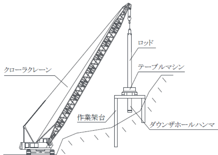
参考図 (C工法模式図)
