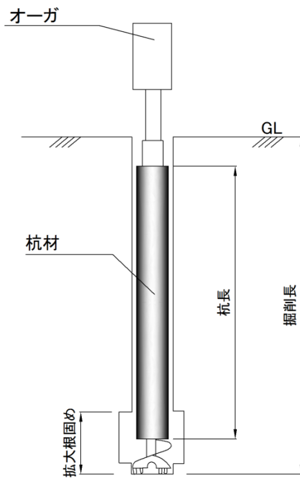
図 1-1 施工図（グラウト注入）
