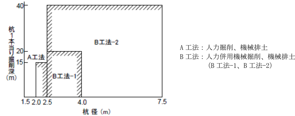
図 1-1 適用杭径及び掘削深（標準）
