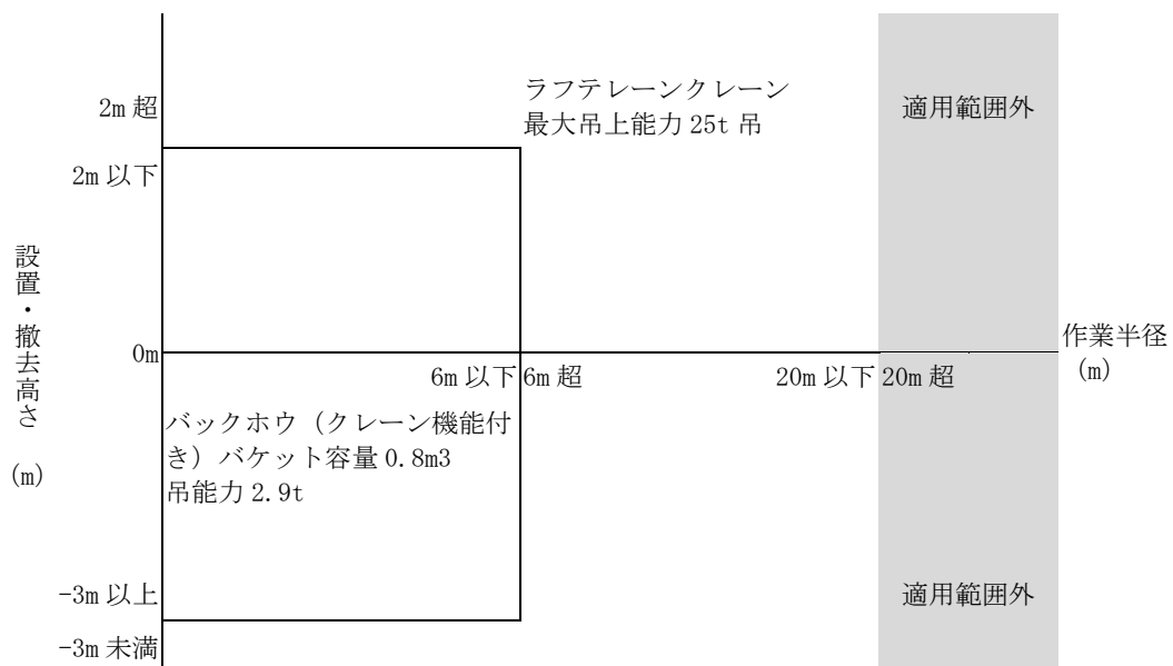
図 3-1 機種選定 製作・設置
