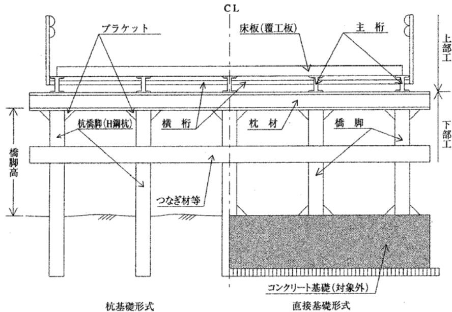
圖 2-2 仮橋・仮棧橋工概念図
