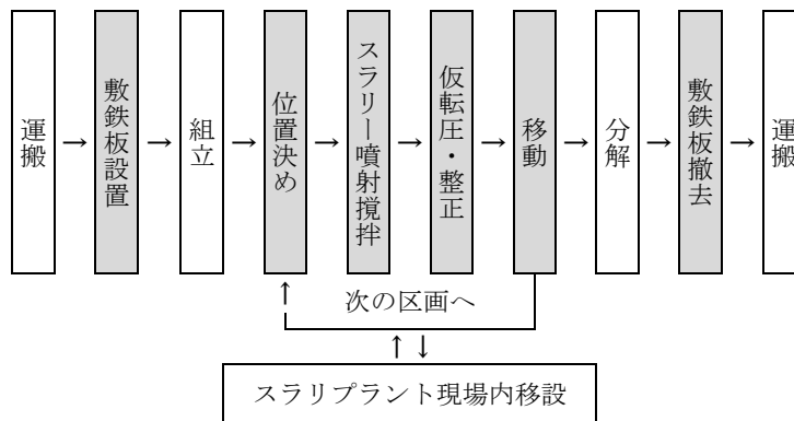
図 2-1 施工フロー
