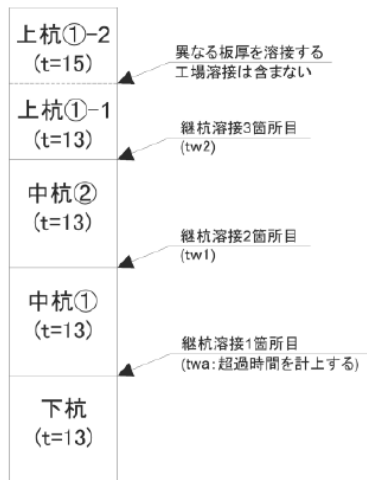
図 5-2 継杭溶接箇所（参考図）
