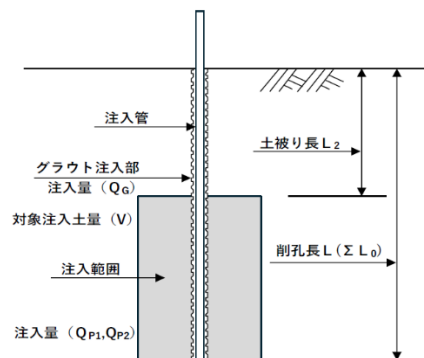
図 3.2 施工図（二重管ダブルパッカー工法）
