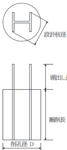
H 形鋼の場合
