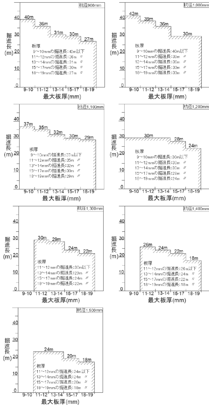
図 1-1 適用掘進長
