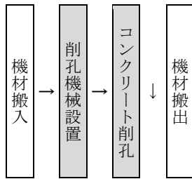
図 2-1 施工フロー
