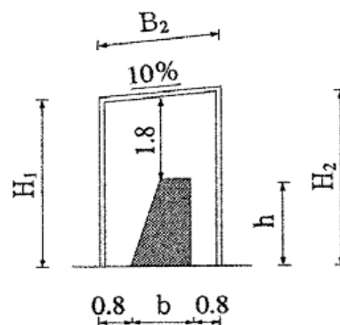
(断面図)
