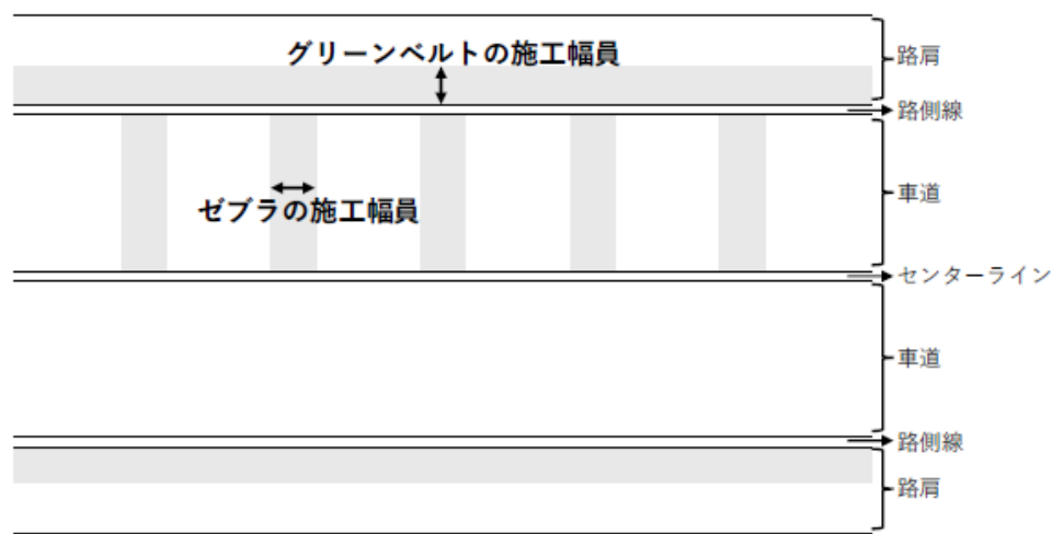
図 2.1 平面模式図
