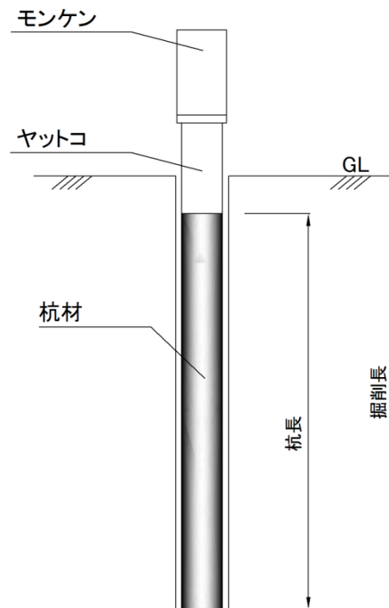
図 1-2 施工図（打撃）
