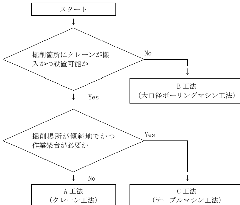
図 2-2 工法の選定
