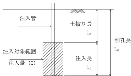
図3-1 施工図
