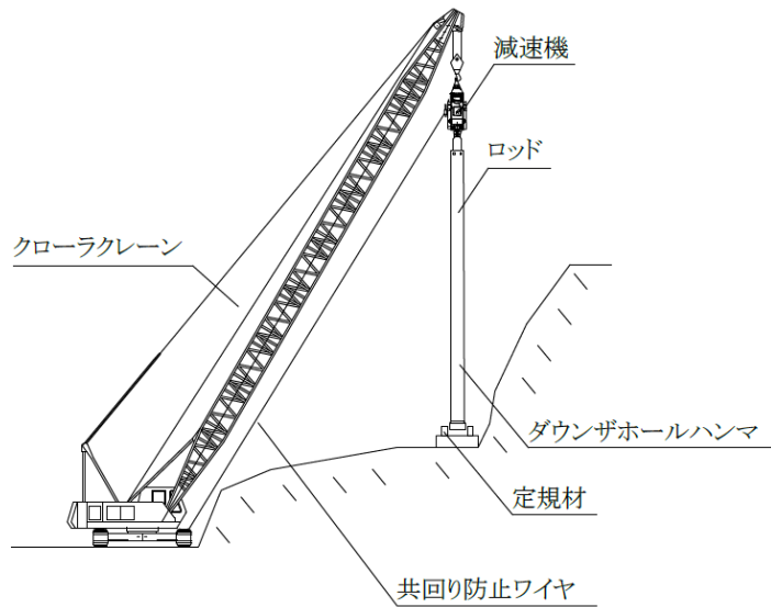
参考図 (A 工法模式図)
