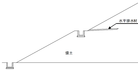
水平排水材の参考図
