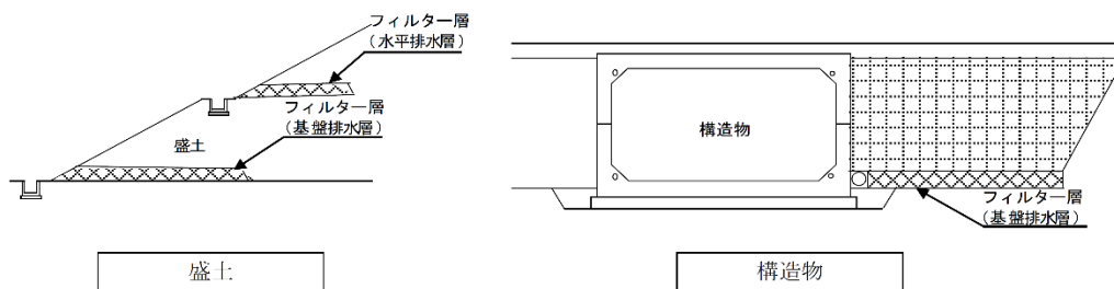
フィルター層の参考図
