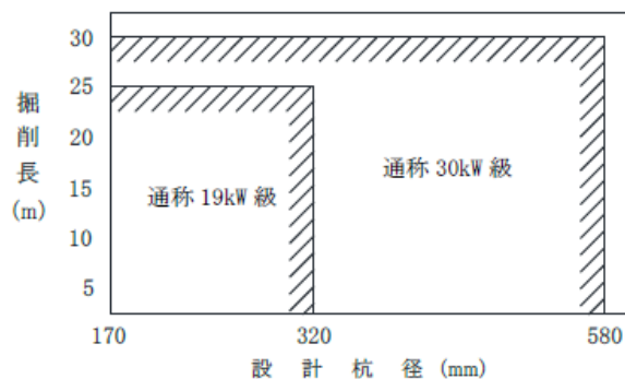
図 3-1 大口径ボーリングマシンの選定
