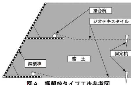
図 A 鋼製枠タイプ工法参考図
