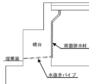
橋台
