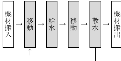
図 2-1 施工フロー
