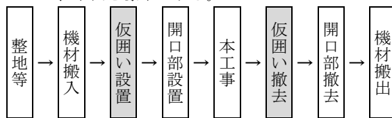
図 2-1 施工フロー
