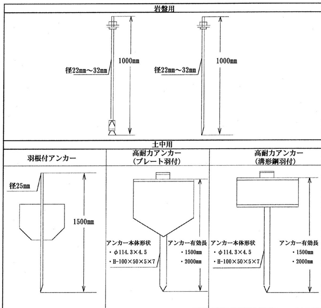
ポケット式支柱（アンカー固定式）
