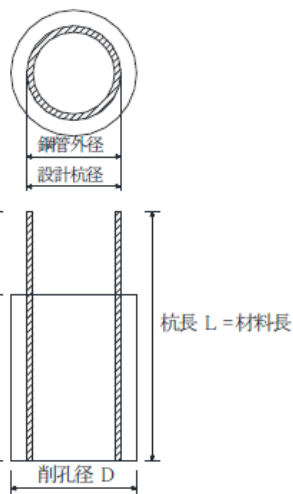
図 1-1 施工図
