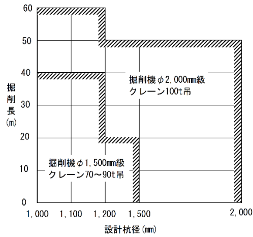
図 3-1 全回転型オールケーシング掘削機とクローラクレーンの選定図
