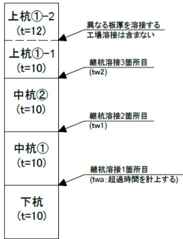
図 5-1 継杭溶接箇所（参考図）
