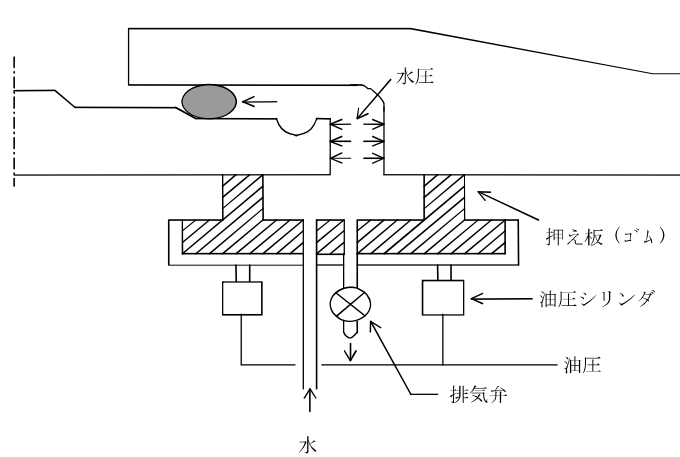
図－３ テストバンドの機構の概略
